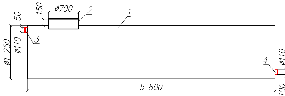
Разрез 1-1
