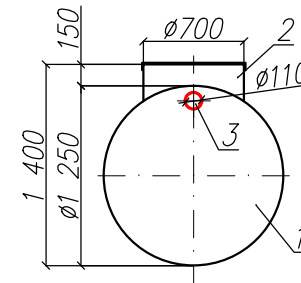
Вид спереди
