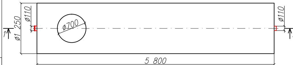
Вид сверху
